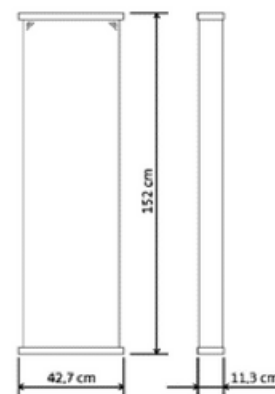
Dimensiones en cm
